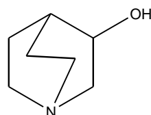
XII. 3-Quinuclidinol [1619-34-7]
